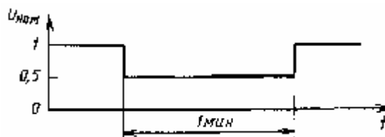
Рисунок 3 — Провалы напряжения \Delta U = 50\%
