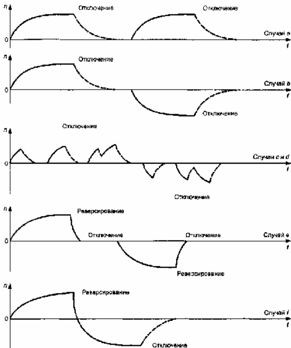
Рисунок 6 — Примеры кривых скорость — время, соответствующие случаям а)–ф) по 4.3.5.5 (пунктирные участки кривых обозначают периоды обесточивания двигателя)
