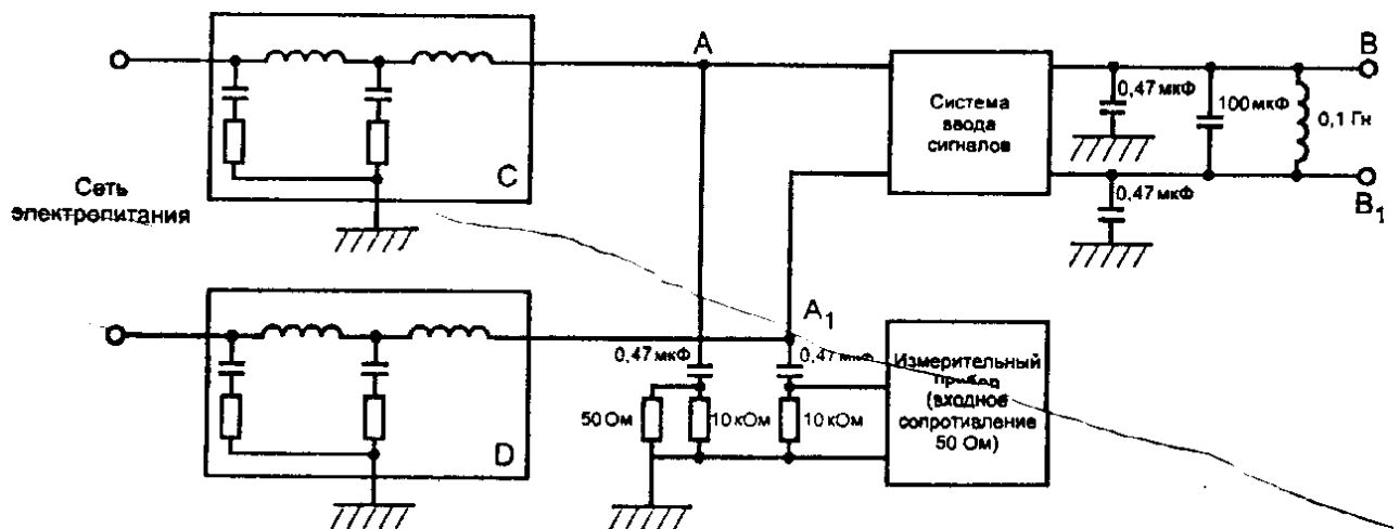
Рисунок 1 - Измерение симметричного напряжения выходных сигналов в полосе частот от 3 до 9 кГц
