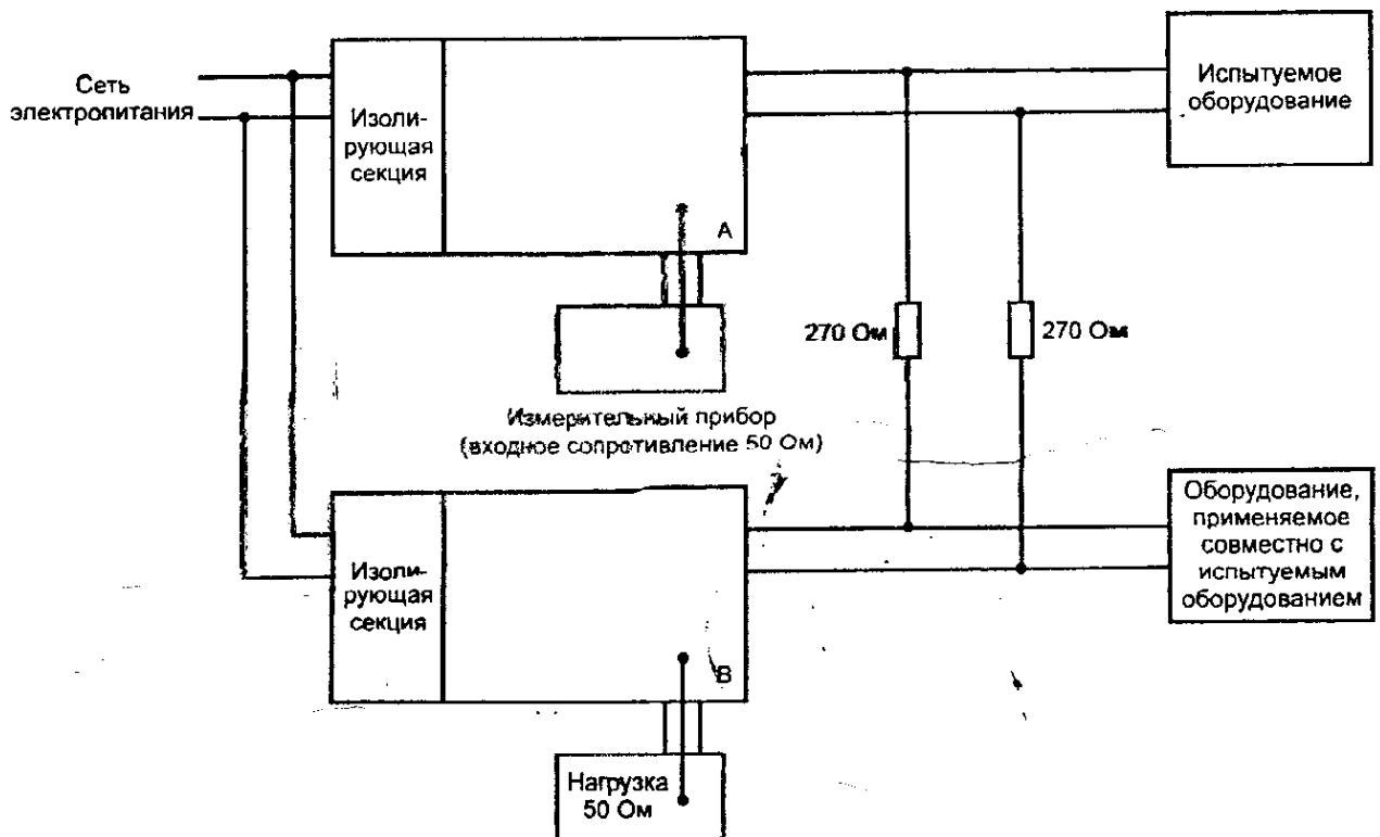
А, В - эквиваленты сети по ГОСТ Р 51319 (типы 1, 4)
