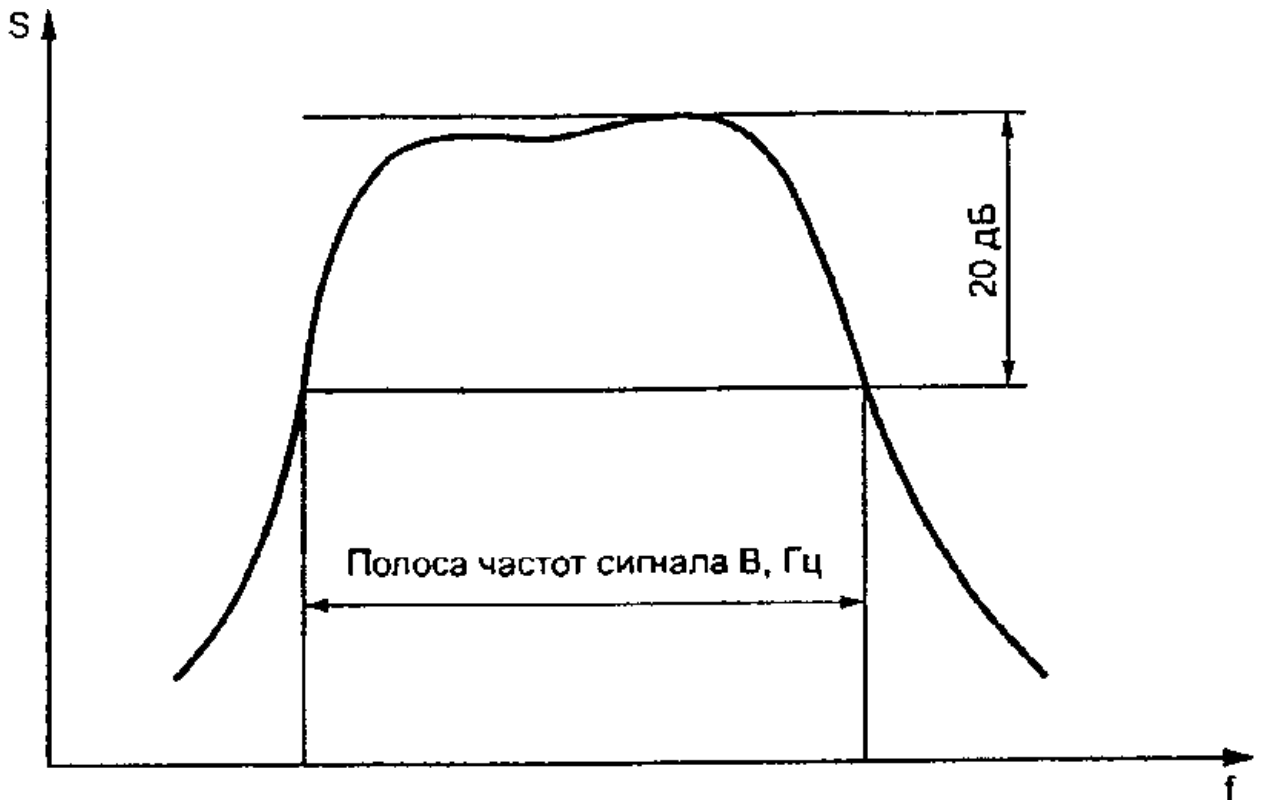
Рисунок 3 - Измерение полосы частот сигнала
