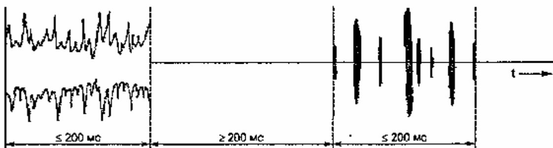
Две кратковременные ИРП Две ИРП длительностью не более 200 мс каждая, разделенные интервалом не менее 200 мс, наблюдаемые на выходе ПЧ измерителя ИРП Рисунок 3в Рисунок 3 Примеры прерывистых ИРП, нормируемых как кратковременные ИРП (см.
