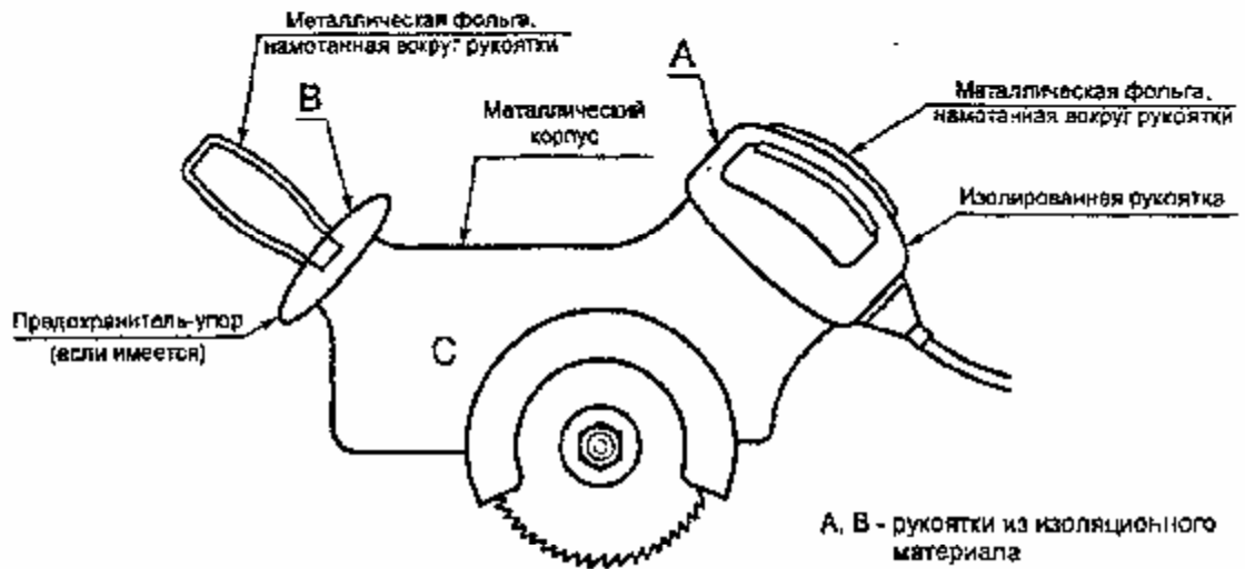
Рисунок 8в — Ручная (портативная) электропила
