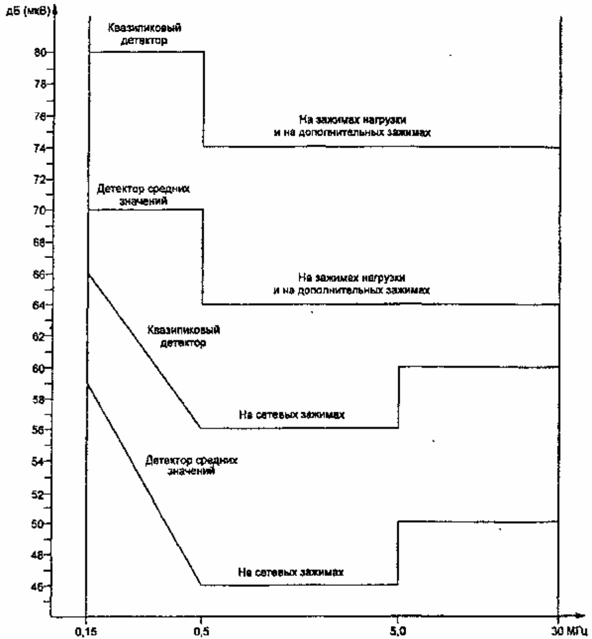
Рисунок 2 — Графическое представление норм (см. 4.1.1)
