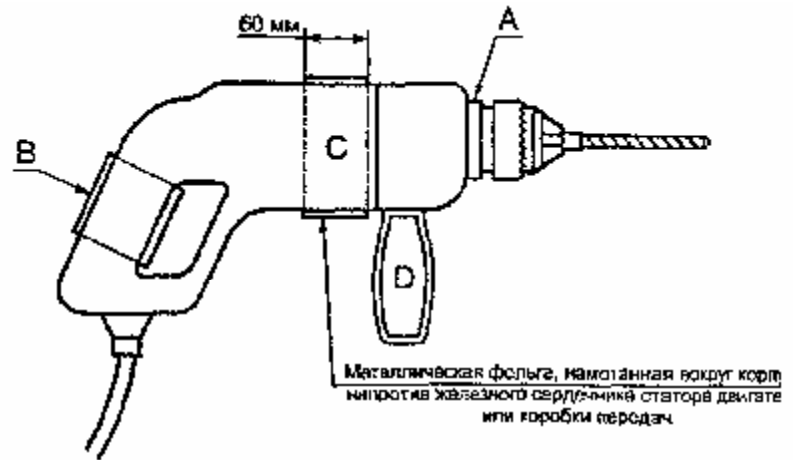
Рисунок 8б — Ручная (портативная) электрическая дрель
