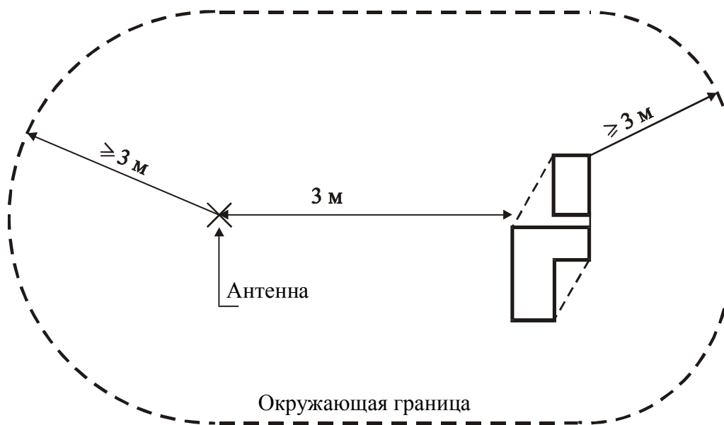
Рисунок 1 - Измерительная площадка
