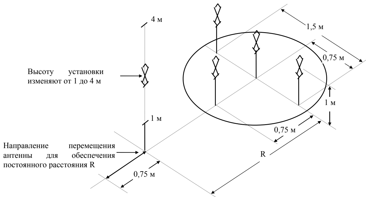
Рисунок Д.3 - Расположения антенн при измерении затухания альтернативной площадки (вертикальная поляризация) для испытываемого объема с размерами не более (1 \times 1,5 \times 1,5) м и при расстоянии от задней границы объема до ближайшей точки конструкции и/или радиопоглощающего материала более 1 м
