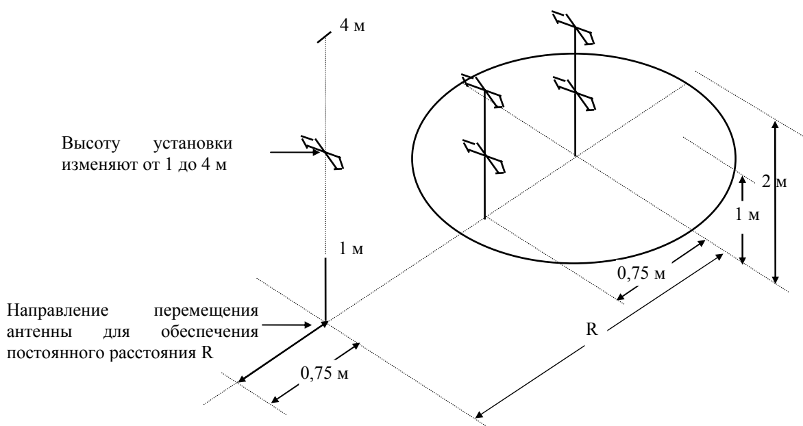
Рисунок Д.4 - Расположения антенн при измерении затухания альтернативной площадки (горизонтальная поляризация) для испытываемого объема с размерами не более (1 \times 1,5 \times 1,5) м и при расстоянии от задней границы объема до ближайшей точки конструкции и/или радиопоглощающего материала более 1 м
