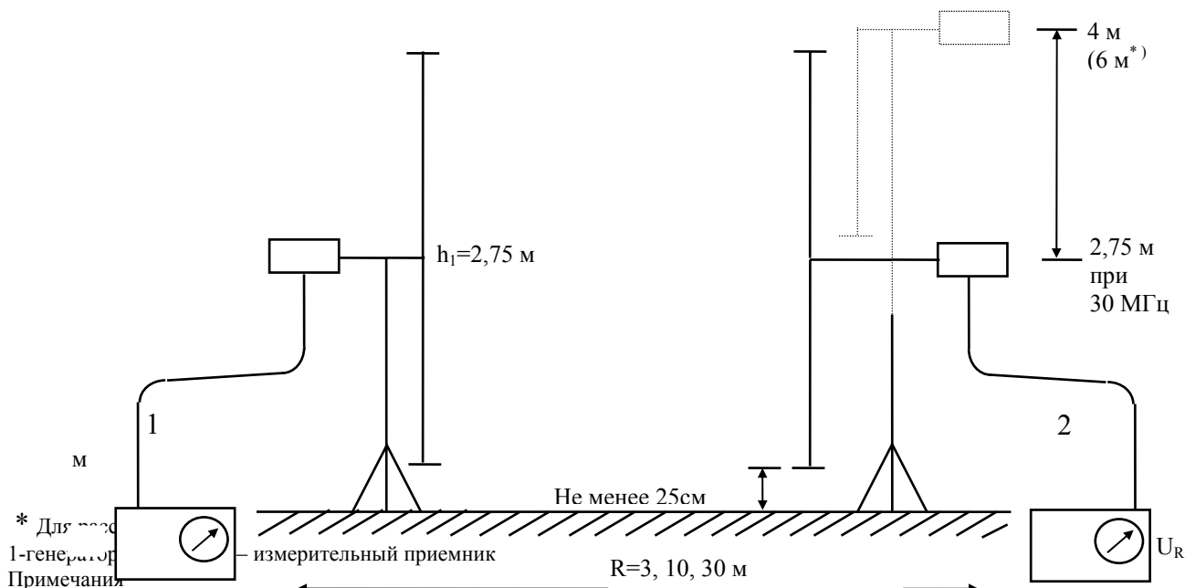
Рисунок Г.2 - Схема измерения затухания площадки при вертикальной поляризации
