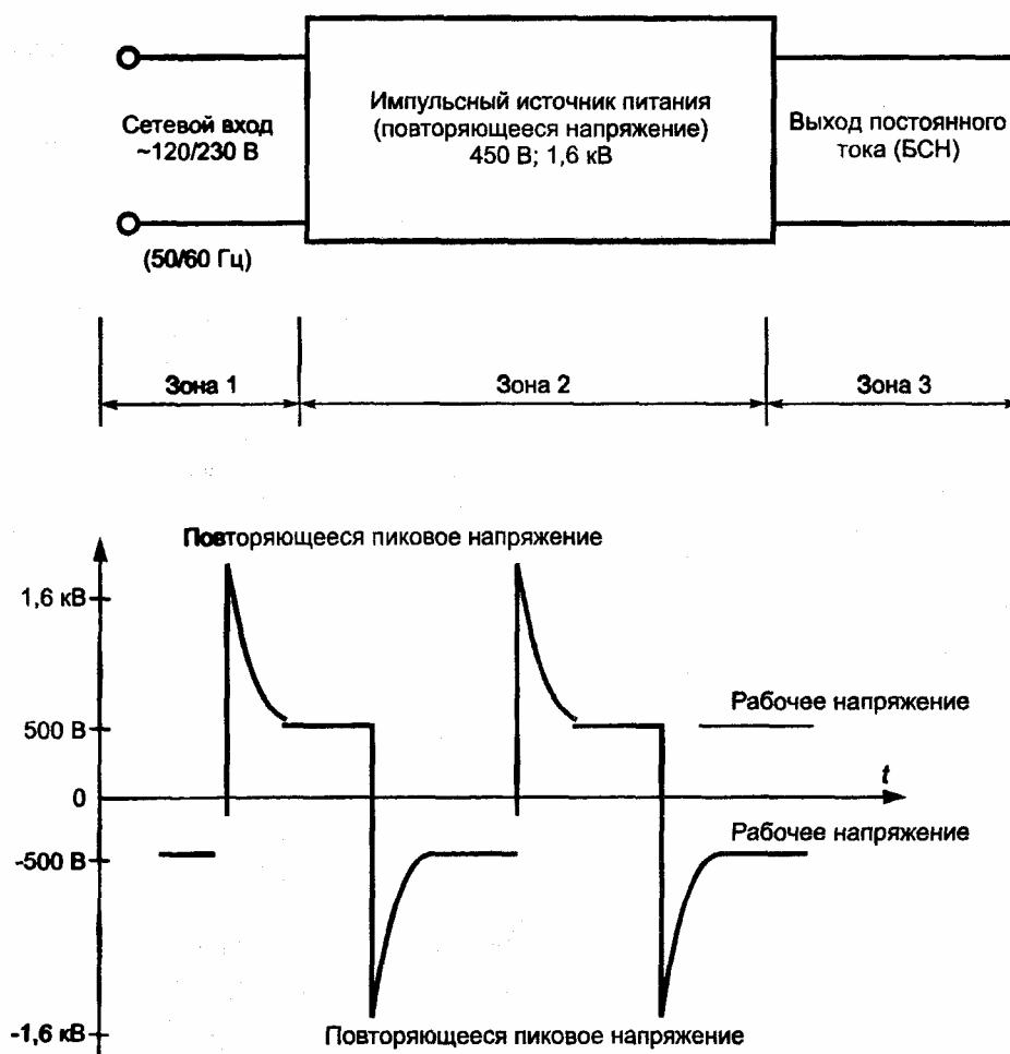
Рисунок Е. 1 — Пути утечки для схем, в которых генерируются повторяющиеся пиковые напряжения
