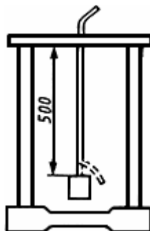
Рисунок 1 - Схема приспособления для испытания шнура на растяжение
