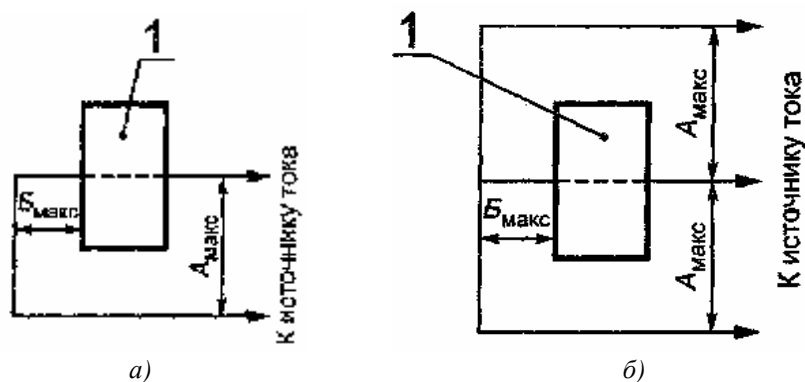
1 — испытываемый трансформатор; A_{\max} — расстояние между осями проводников соседних фаз в месте установки трансформатора в эксплуатации; — расстояние в свету от трансформатора до места ближайшего изгиба проводника, служащего в эксплуатации первичной обмоткой трансформатора
