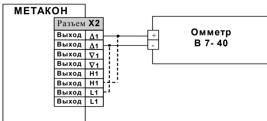
Рис. П.7.1. Схема проверки выходов реле
