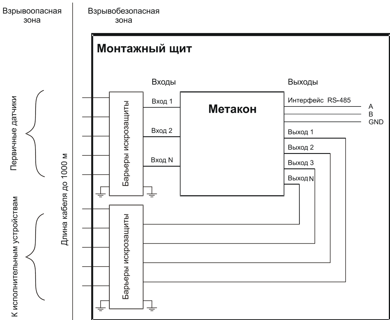
Функциональная схема подключения приборов Метакон при использовании на взрывоопасных производствах
