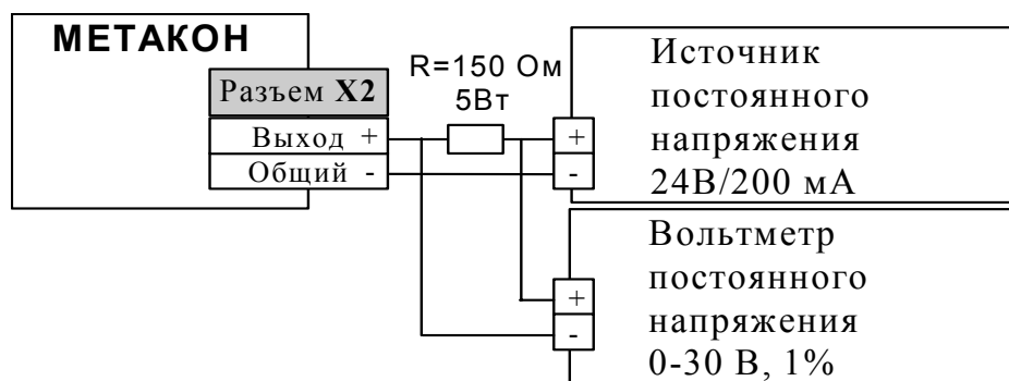
Рис. П.7.2. Схема проверки ключей в выключенном состоянии
